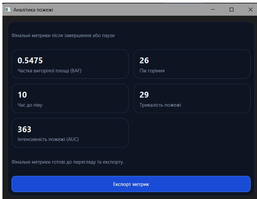
Рисунок 3.11 — Вікно з фінальними метриками
