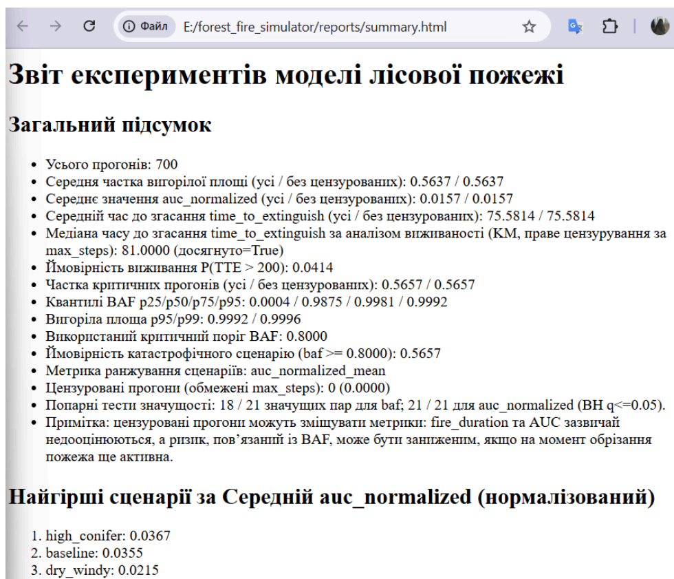
Рисунок 3.14 — Фрагмент згенерованого HTML-звіту із загальним підсумком
