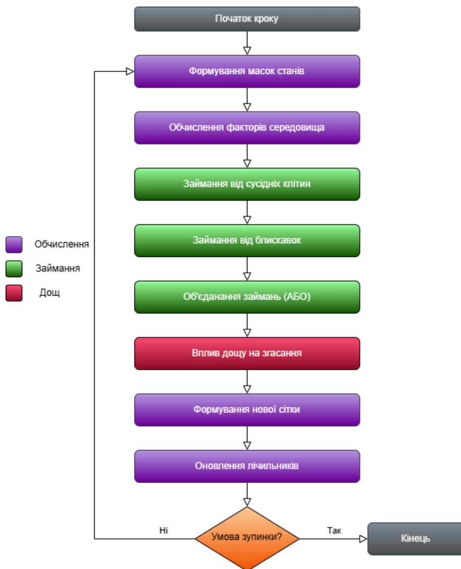
Рисунок 2.1 Схема одного кроку симуляції
