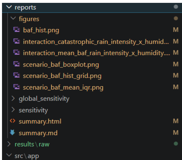
Рисунок 3.13 — Структура згенерованих файлів звіту
