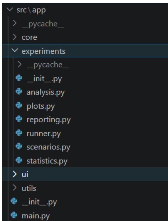
Рисунок 3.4 — Структура шару experiments
