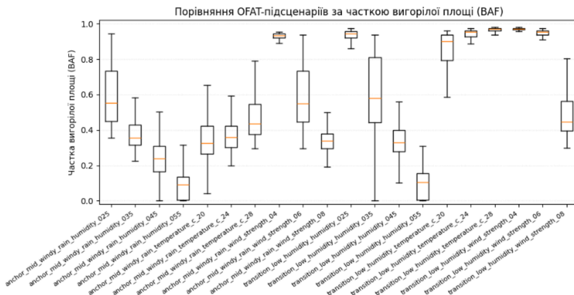
Рисунок 3.16 — Порівняння OFAT-підсценаріїв за часткою вигорілої площі BAF
