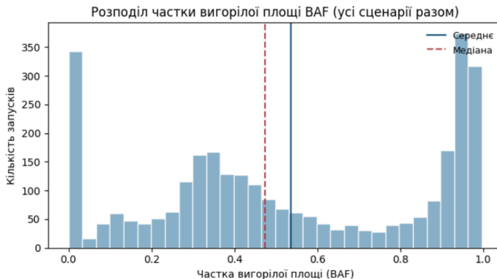
Рисунок 3.15 — Гістограма розподілу частки вигорілої площі BAF
